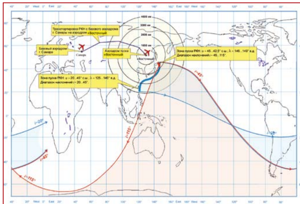
Схема полета системы «Воздушный старт» с космодрома «Восточный»
