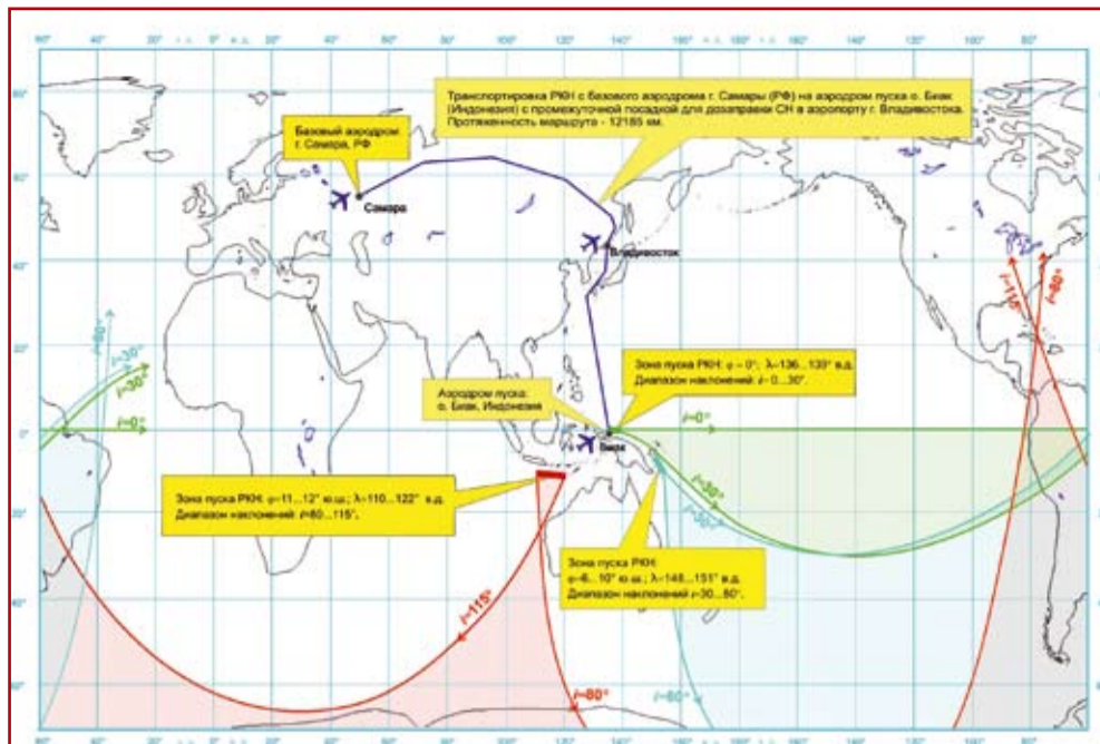
Схема полета системы «Воздушный старт» с космопорта Frans Kaisiepo (о.Биак)
