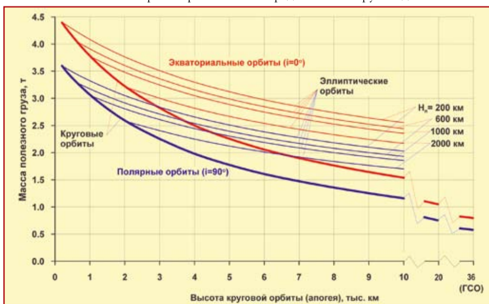
Энергетические возможности системы «Воздушный старт»
