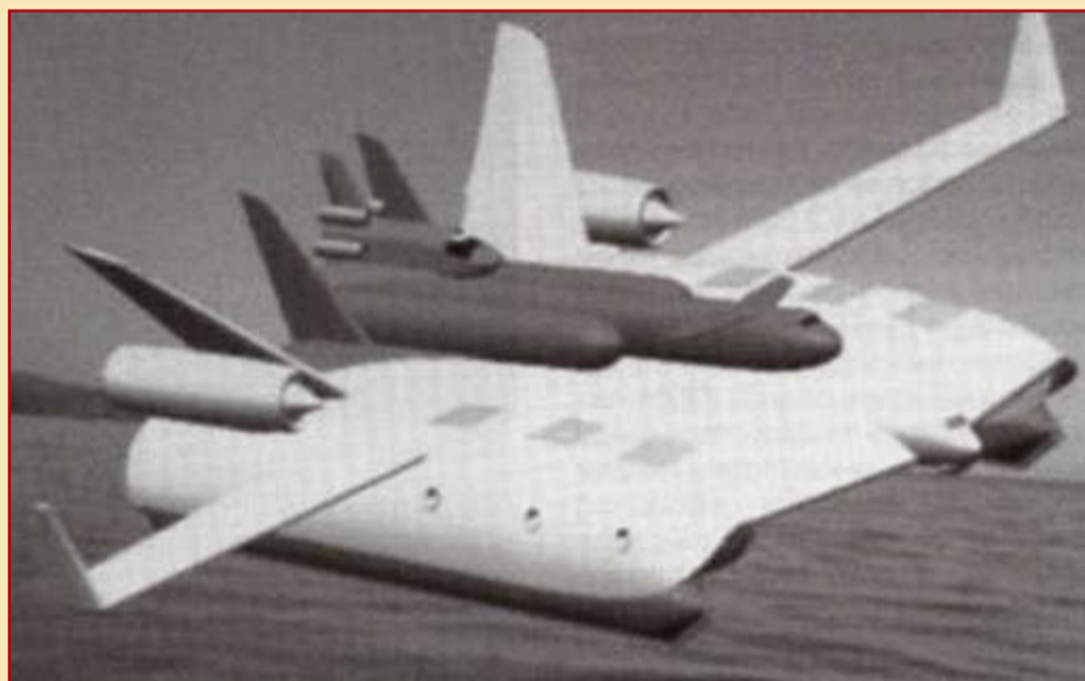
Проект «Бе 2500 - Нептун»
