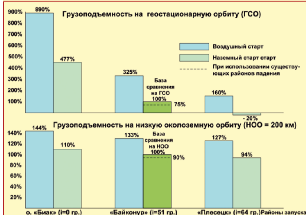
Сравнение грузоподъемности ракет-носителей наземного и Воздушного стартов при выведении на низкие и геостационарную орбиты
