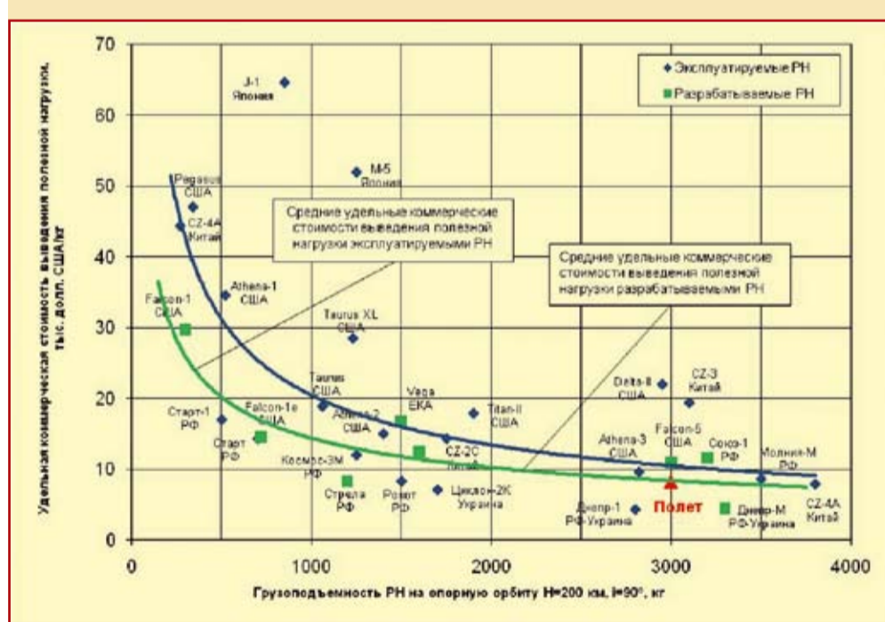
Удельная коммерческая стоимость выведения полезной нагрузки на низкую опорную орбиту H=200 км, i=90°
